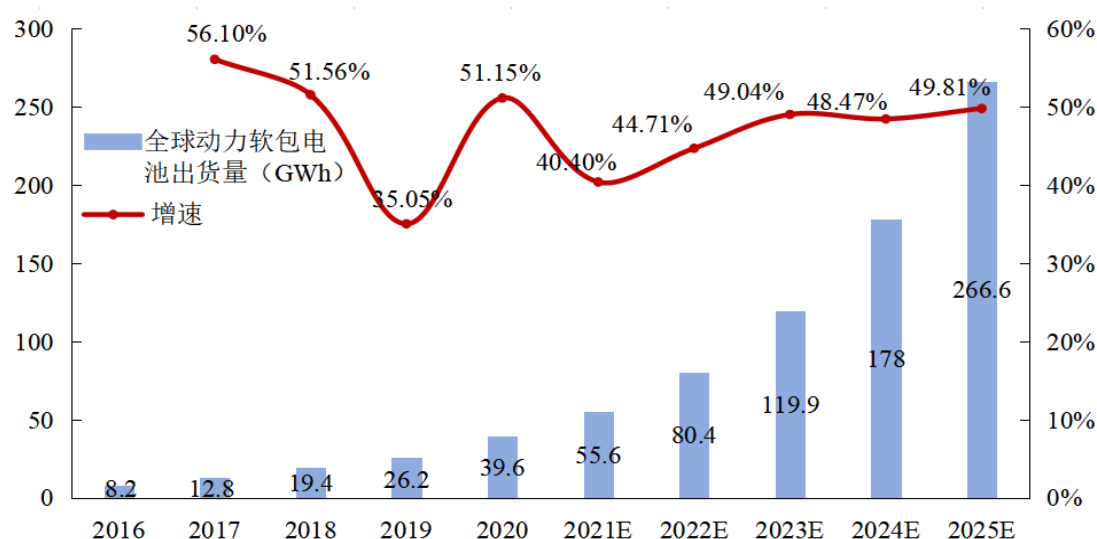
2016-2020 年全球动力软包电池出货量以及 2021-2025 年预测出货情况
