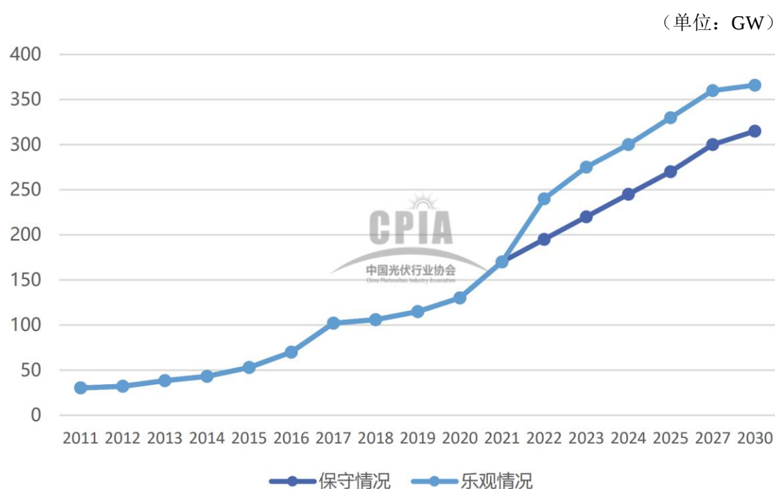
2011-2021 年我国光伏年度新增装机规模以及 2022-2030 年新增规模预测
