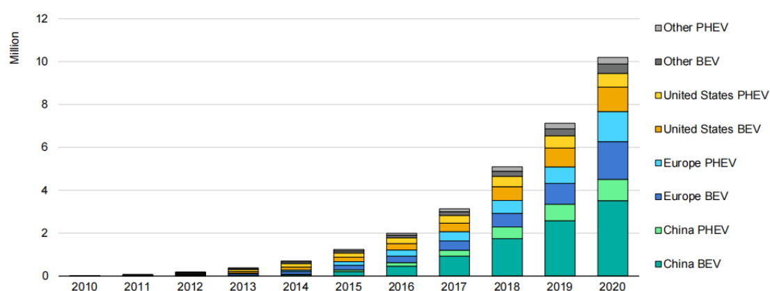
2010-2020 年全球新能源汽车保有量变化情况
